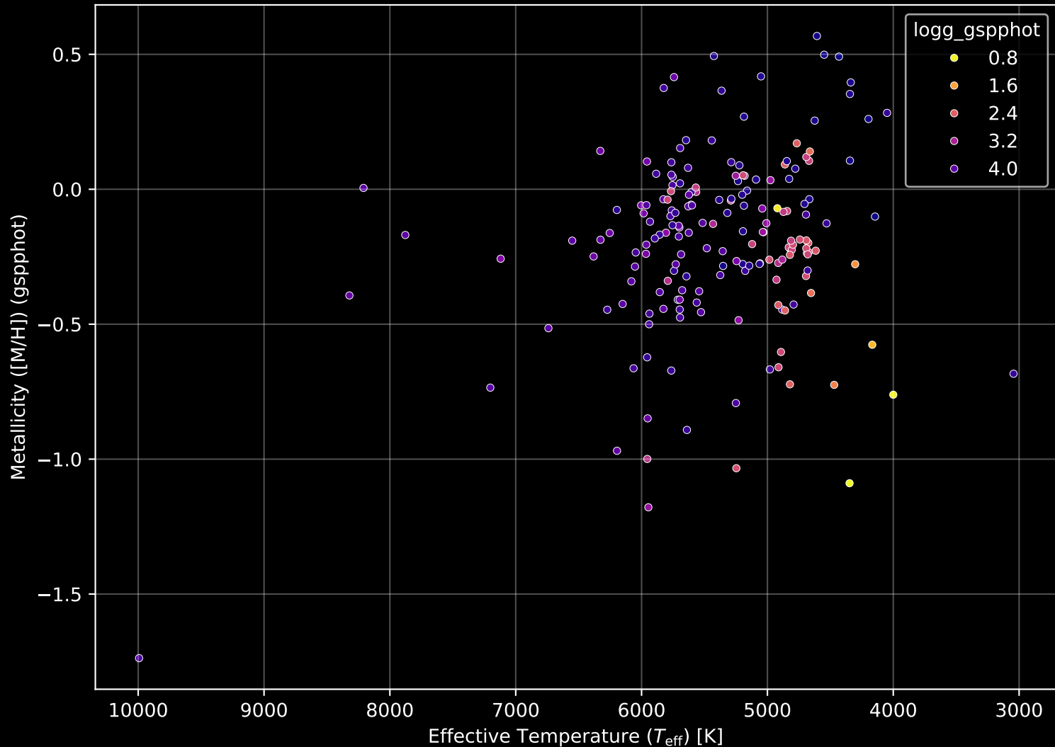
APOGEE DR17 Field: [269-30-O_TESS] Stellar Population Parameters (n= 183)
